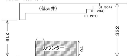
入口付近 断面図
