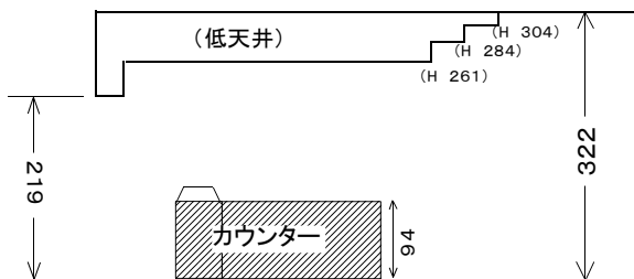
入口付近 断面図
