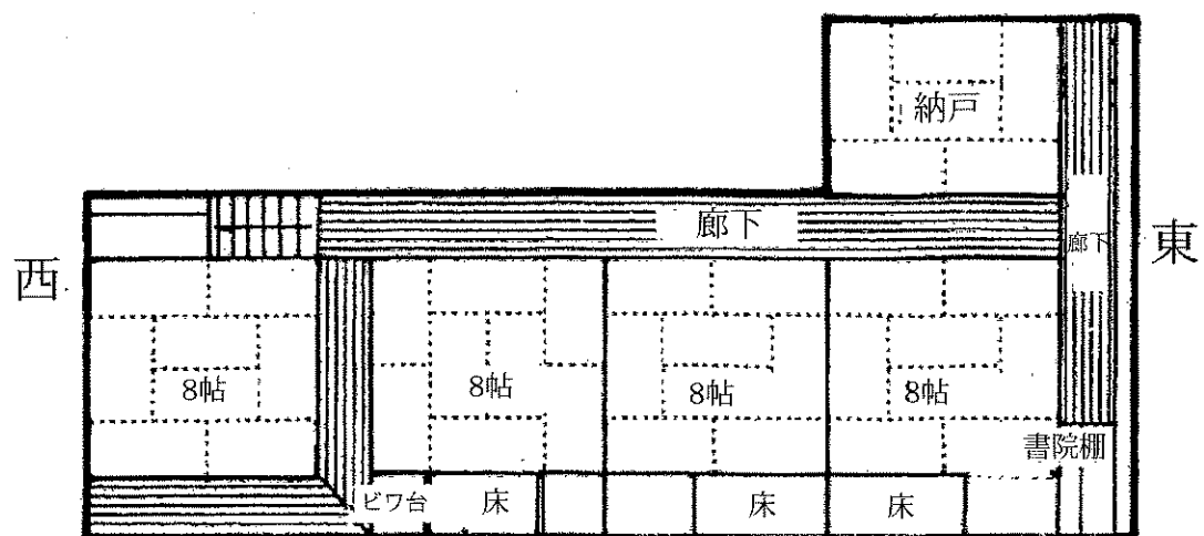
2階平面図
